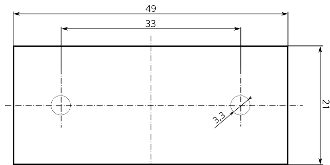
Bohrplan Goblin-EXP
